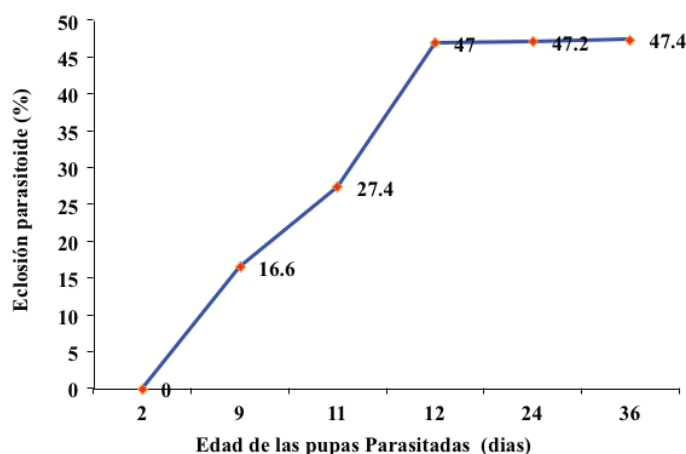
Figura 17. Eclosión de parasitoide para mosca del establo según edad de pupas de cría. INTA 2011.
