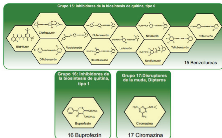
Figura 18. Insecticidas inhibidores de crecimiento de estadios de mosca del establo y otros dípteros. IRAC Feb 2012 ( www.irac-online.org ).
