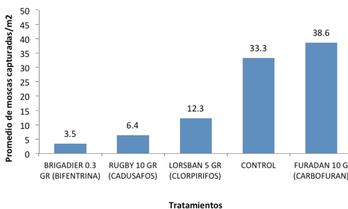
Figura 20. Adultos de mosca del establo según insecticidas larvicidas aplicados en rastrojos de piña con larvas. PINDECO 2012.
