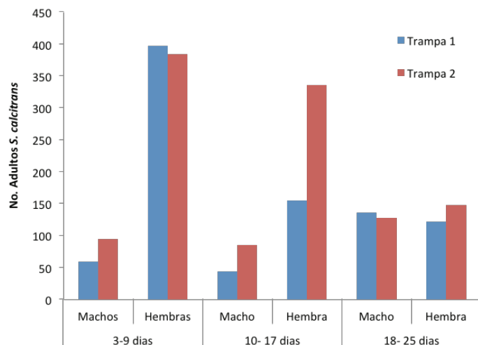
Figura 11.- Proporción macho hembra de mosca del establo S. calcitrans según edad del rastrojo de piña en derriba en verde. INTA/Pindeco. Feb—Mar 2013.
