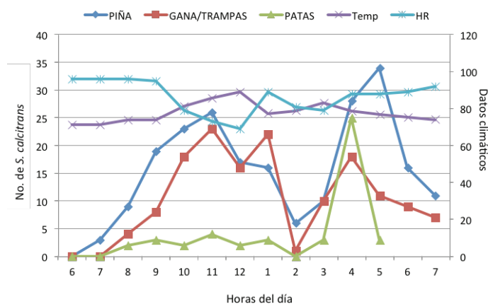
Figura 9b. Actividad diaria de mosca del establo S. calcitrans en los establos de la ganadería semiestabulada, las patas de los animales y Piñera en Verano . INTA, 2012
