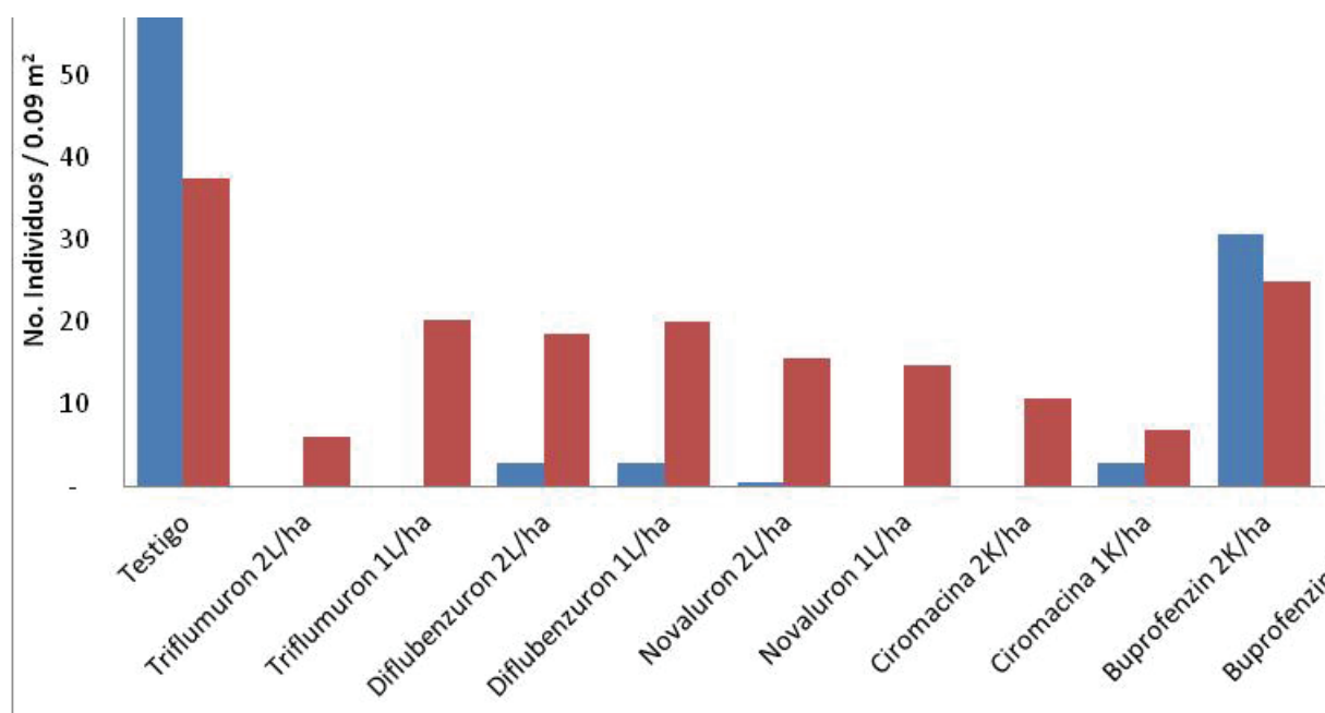
Figura 19. Control químico de mosca del establo según insecticida. INTA 2013
